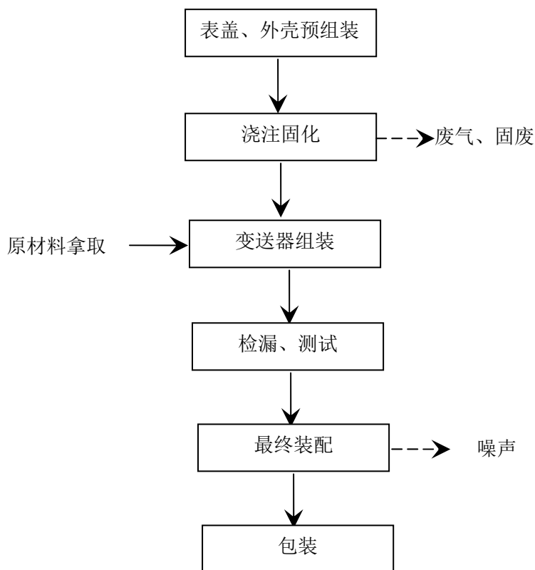
图 2-1 压力变送器工艺流程和产污环节图
