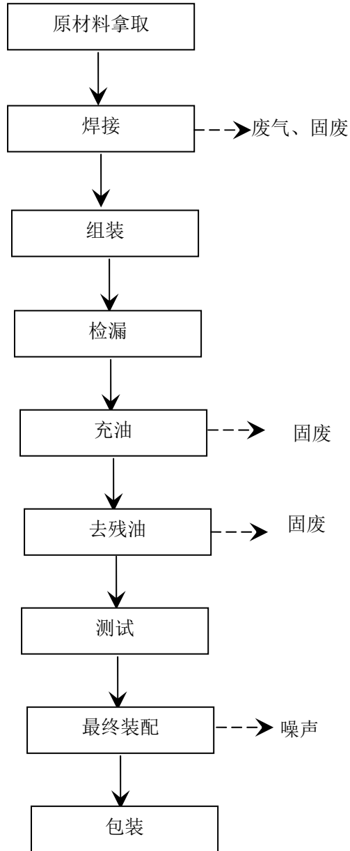
图 2-3 差压液位工艺流程和产污环节图
